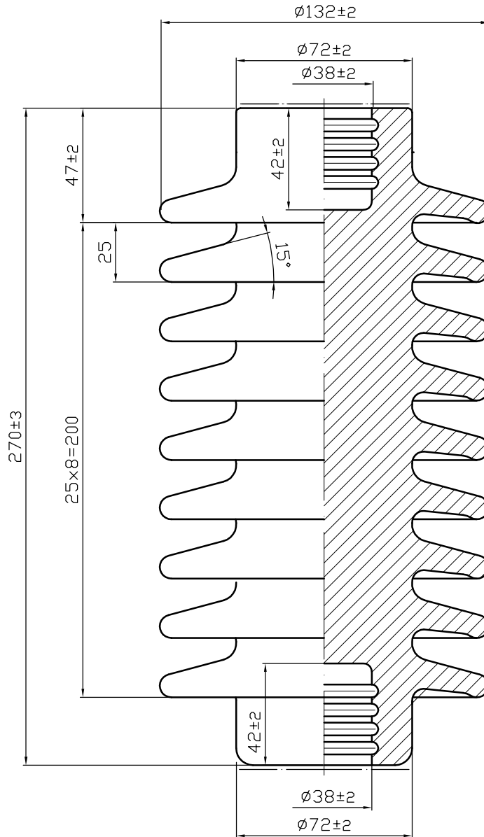
SÚ CẦU CHÌ 15KV(SCR15.TK) 15KV PUSE CUT-OUT INSULATORS (SCR15.TK)
